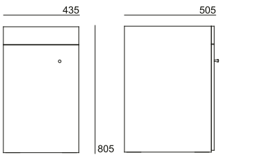
Móvel Mozela . Mueble Mozela . Mozela furniture . Meuble Mozela 55332010
