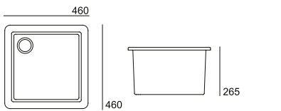
Pia Monchique . Pila Monchique . Monchique Sink . Évier Monchique 78618XX2C
