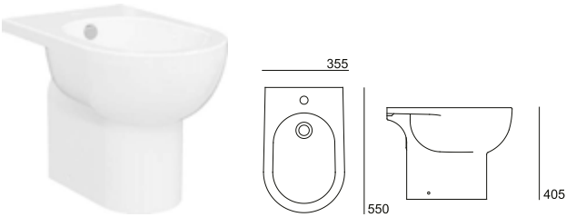
Bidé . Bidet 37411XX2K
